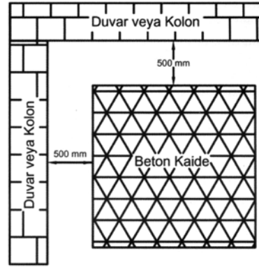
Kaide Betonuna Üst Görünüşü
